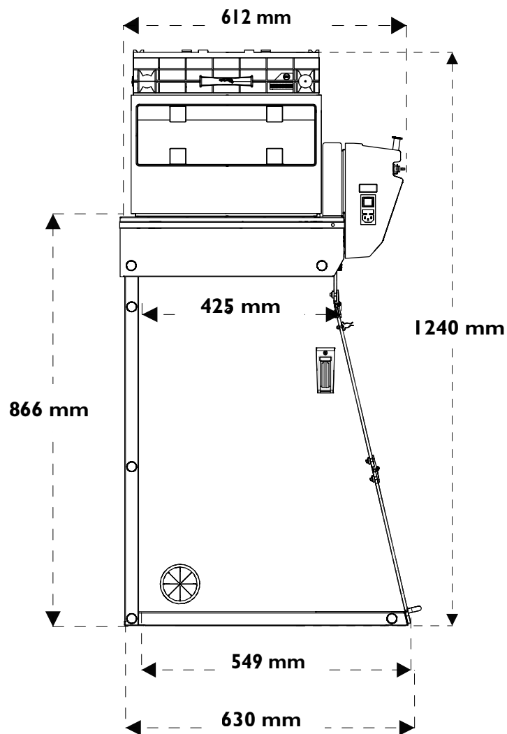
Schema della versione equipaggiata della colonna di filtrazione IP1C
